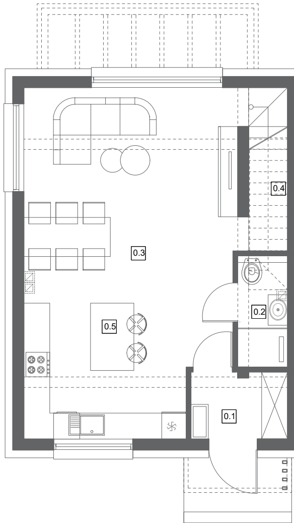
RZUT PARTERU
