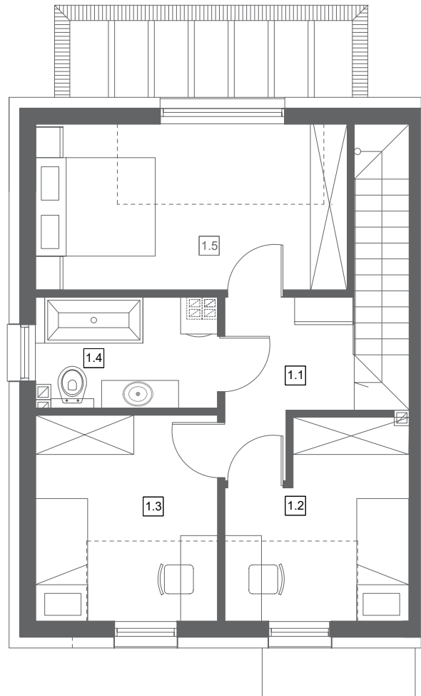
RZUT PODDASZA
