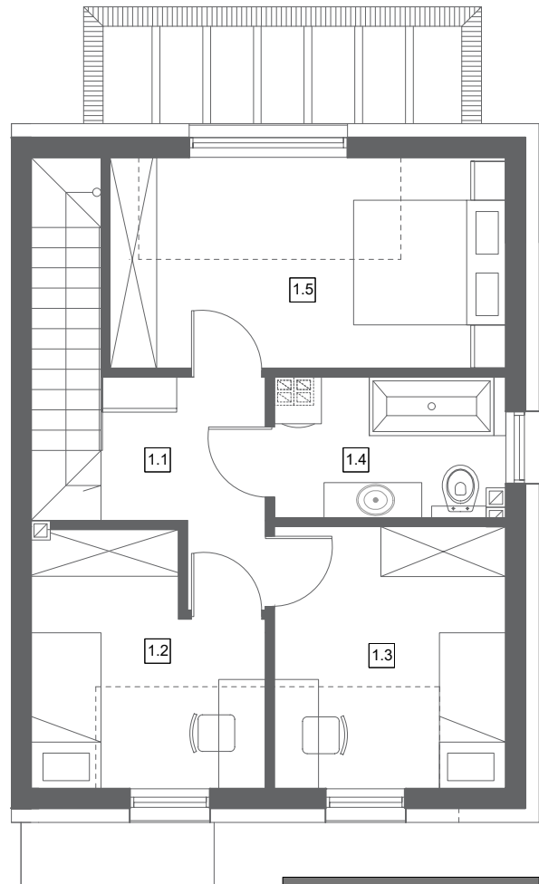
RZUT PODDASZA
