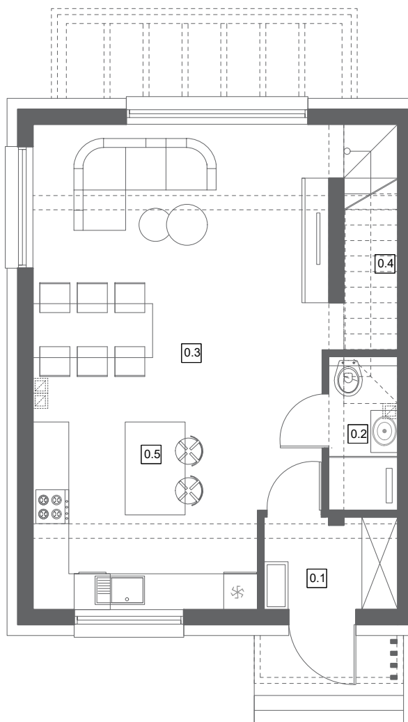
MIESZKANIE 12- PARTER -44,04 m 2
